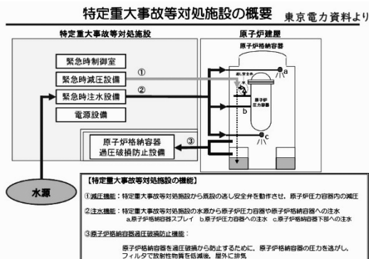
柏崎刈羽原発の特定重大事故対処等施設の例
