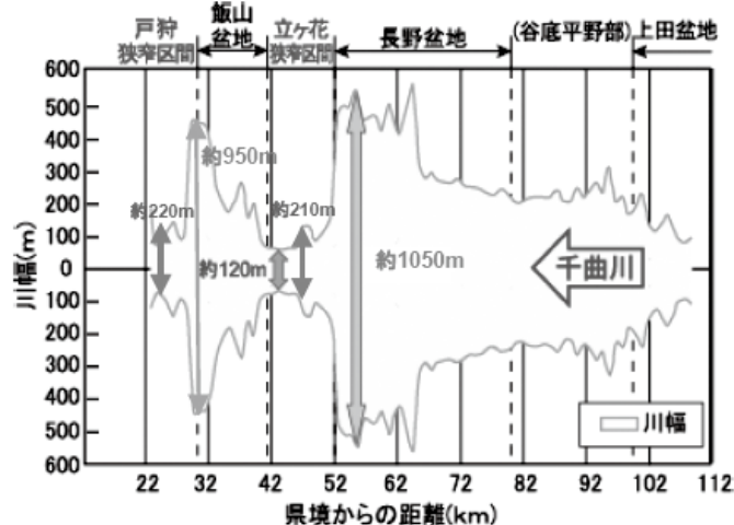
図：千曲川の川幅
